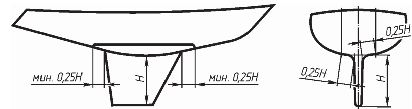
Рис. 3.1.7 Район крепления киля
